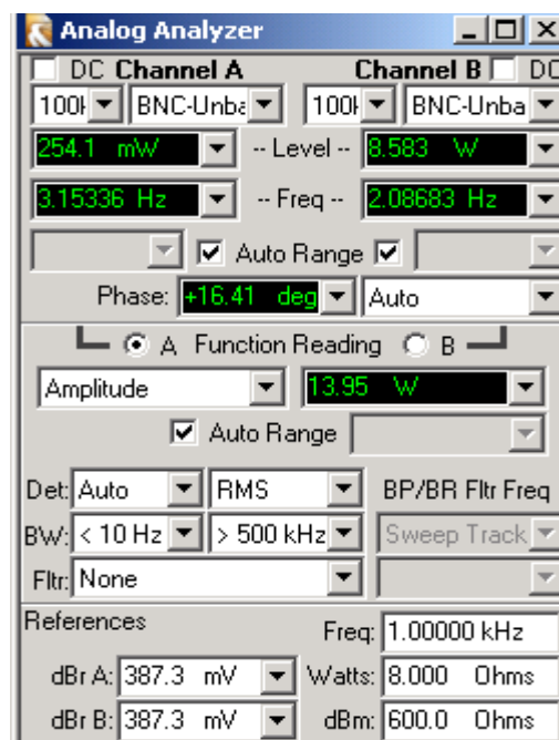
Rys.6. Ustawienia w panelu Analog Analyzer.
