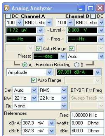
Rys.8. Ustawienia w panelu Analog Analyzer podczas pomiarów stosunku sygnał-szum.
