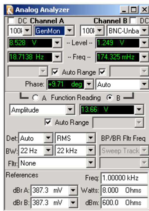
Rys.13. Ustawienia w panelu Analog Analyzer podczas pomiarów przesunięcia fazy wejście/wyjście.
