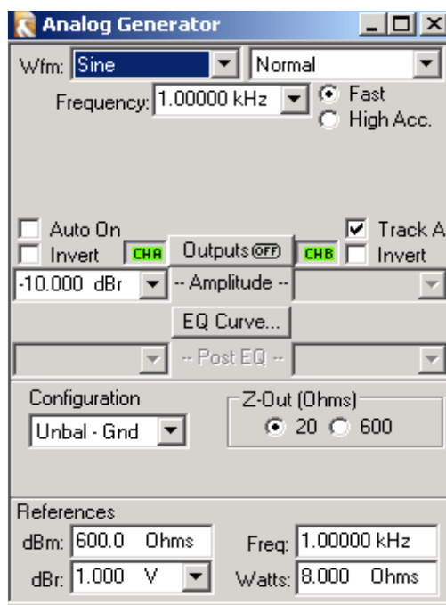
Rys.10. Ustawienia w panelu Analog Generator dla normalnych warunków pomiarowych.
