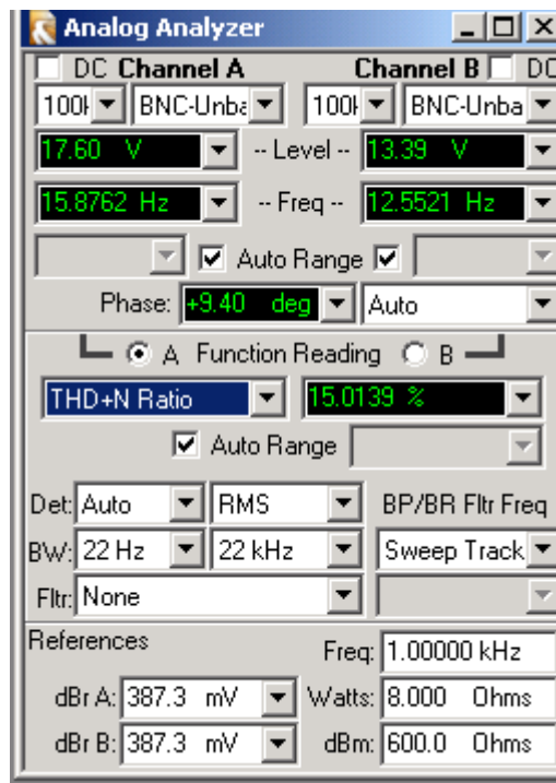
Rys.11. Ustawienia w panelu Analog Analyzer podczas pomiarów całkowitego współczynnika zniekształceń harmoniczných.
